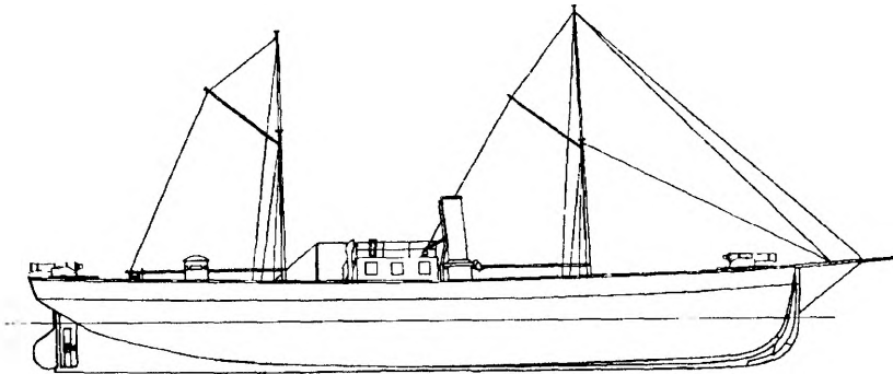
Канонерская лодка типа «Щит». 1855 г. Такие канонерки специально строились для защиты финских шхер в 1854-1855 гг.
