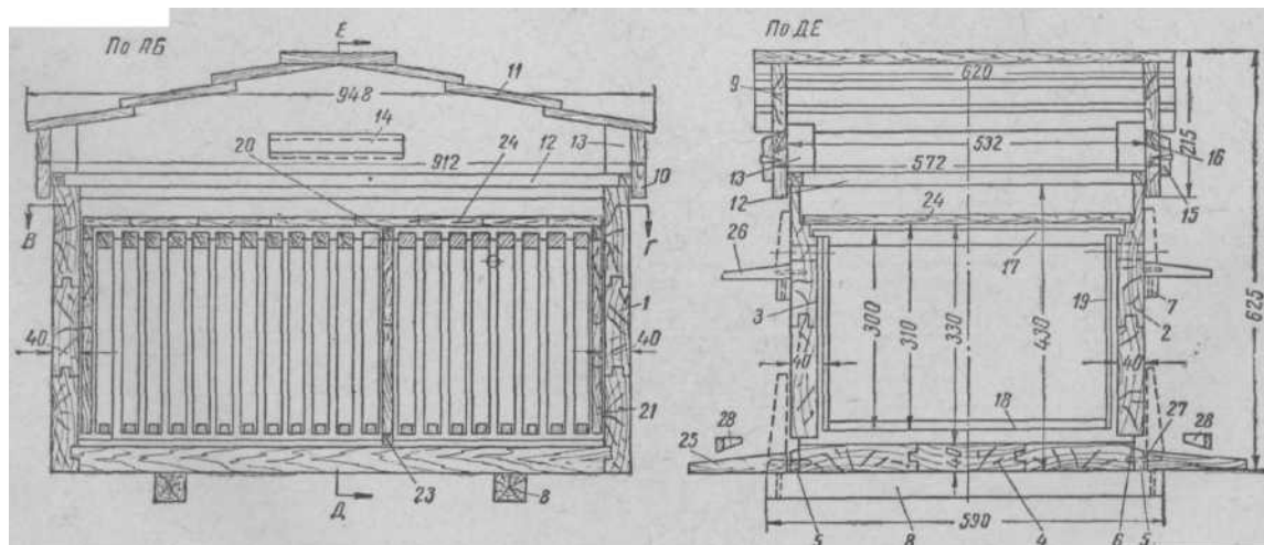
Рис. 6. Размеры улья-лежака.
