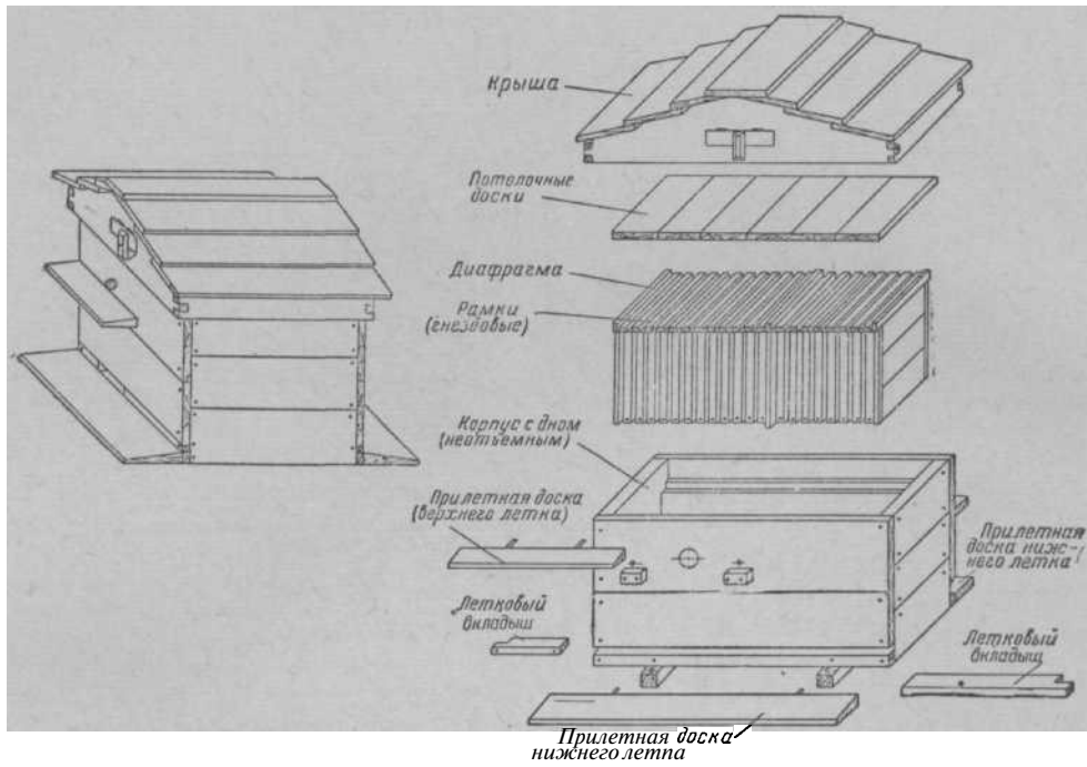
Рис. 3. Одностенный улей-лежак на 20 рамок (общий вид и детали устройства).
