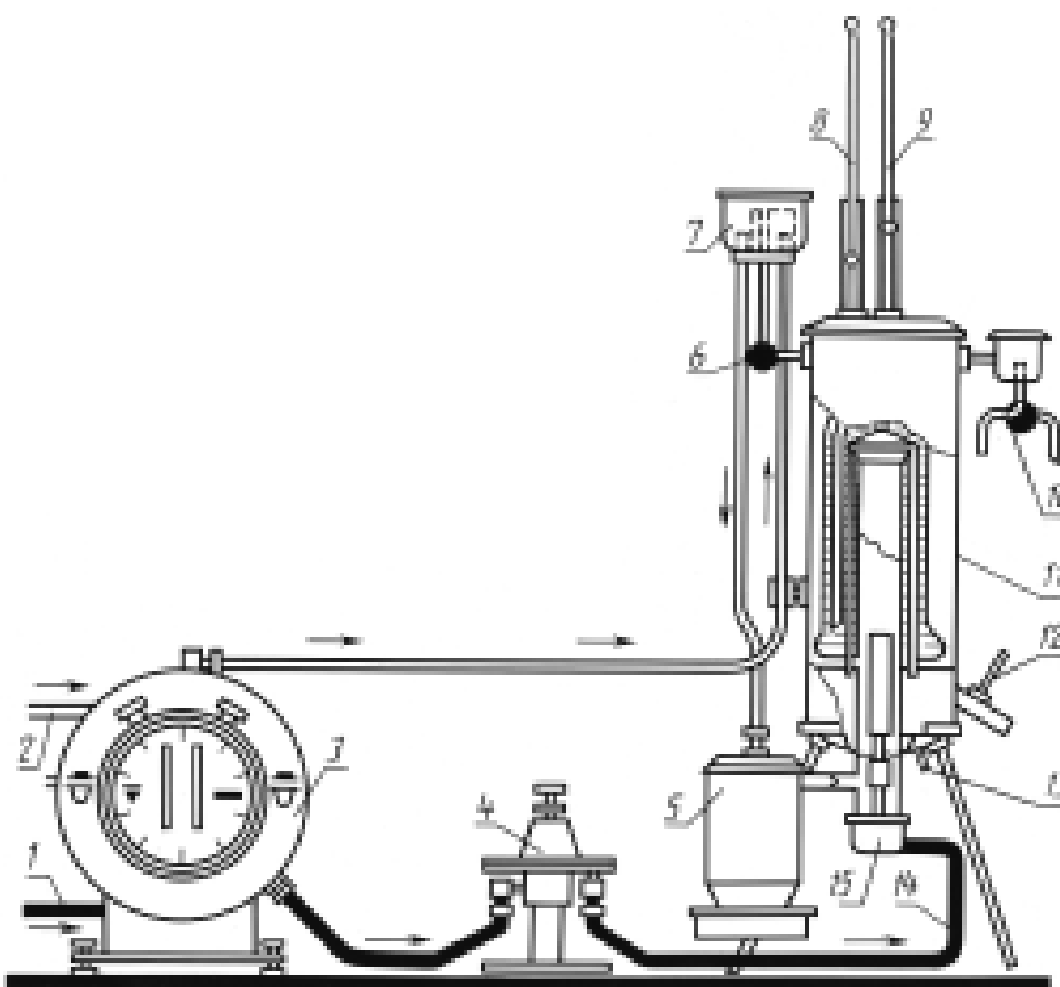
1 — газоподвод; 2 — водопровод; 3 — газовый счетчик; 4 — мембранный регулятор давления высокой чувствительности; 5 — увлажнитель воздуха; 6 — вентиль для регулирования воды; 7 — переливной бак для воды; 8, 9 — термометр для измерения температуры воды на выходе; 10 — трехходовый кран для нагретой воды; 11 — теплообменник; 12 — термометр для измерения температуры отходящих газов; 13 — выпускной патрубок конденсата; 14 — шланг газовой горелки; 15 — газовая горелка
