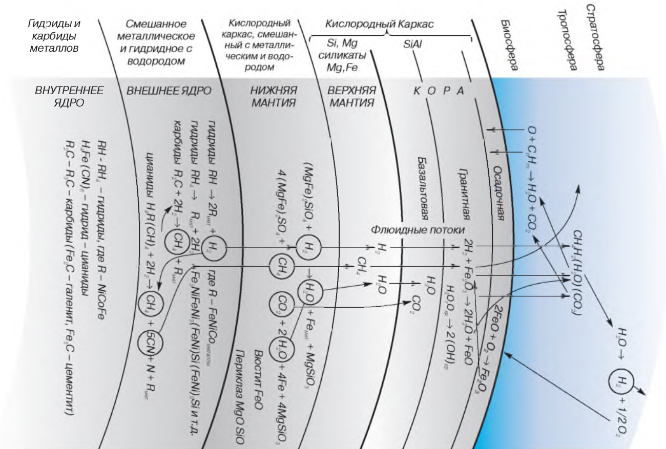
Рис. 1.2. Геохимическая модель Земли
