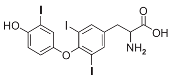
3,3',5'-трийодтироинин — T 3
