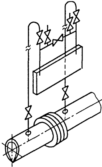
Рисунок В.1 - Дифманометр над трубопроводом
