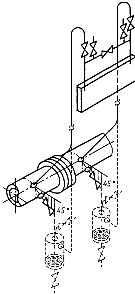
Рисунок В.11 - Дифманометр над трубопроводом (два варианта)
