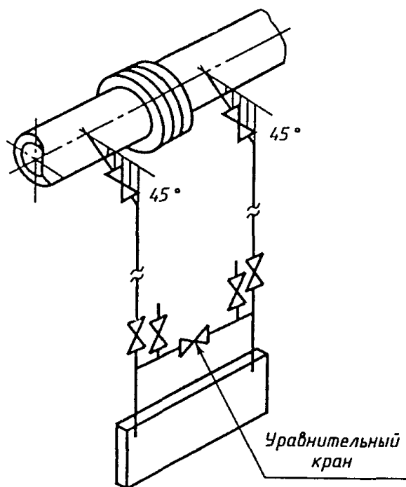
Рисунок В.15 - Дифманометр под трубопроводом
