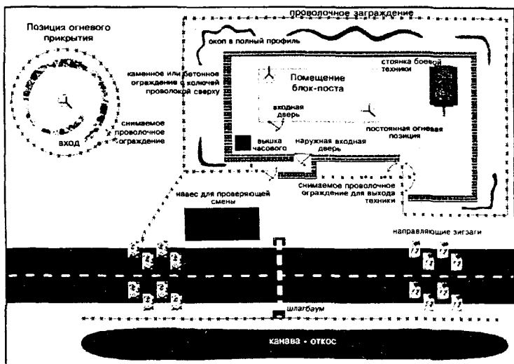
Схема 64. Примерное обустройство фильтрационного блок-поста
