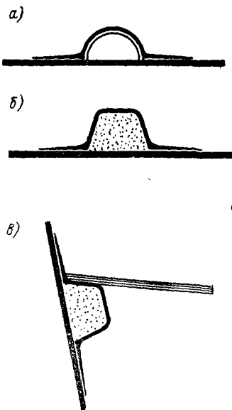
Рис. 127. Конструкции стрингеров.
