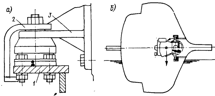
Рис. 177. Ограничитель амортизатора (а) и схема для расчета прочности крепления двигателя к фундаменту (б).
