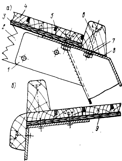
Рис. 105. Два варианта соединения деревянной палубы с металлическим корпусом: а — для яхты «Секура» с надстройкой-баком; б — для гладкопалубной яхты.
