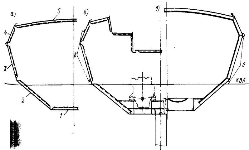
Рис. 96. «Мидель-шпангоут» яхты «Гидра» упрощенной конструкции: а — промежуточный шпангоут; б — сечение по кокпиту; в — рамный шпангоут. 1 — днищевой лист обшивки; 2 — скуловой пояс; 3 — ширетрек (дековой пояс); 4 — комингс бака; 5 — палуба; 6 — монтажные ребра жесткости из угольника.
