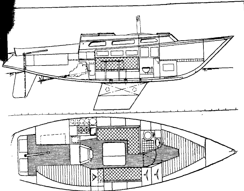
Рис. 52. Схема общего расположения яхты «Гласер-34».
