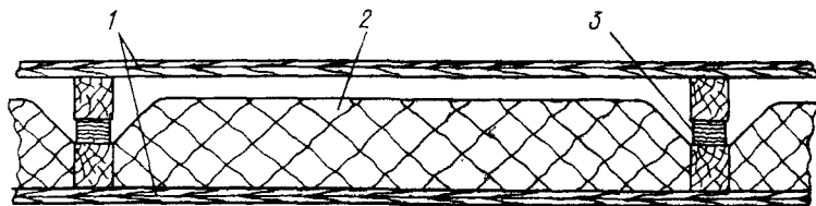
Рис. 148. Легкая переборка с шумопоглощающей изоляцией.
