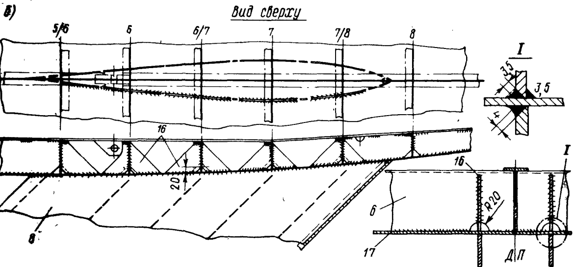
Рис. 101 Сварной киль яхты „Таранга“: а — вариант крепления к днищу на болтах; б — вариант крепления с помощью сварки.
