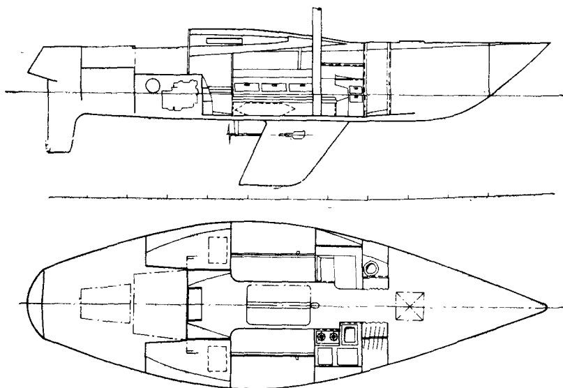
Рис. 38. Схема общего расположения однотонника «Идра».
