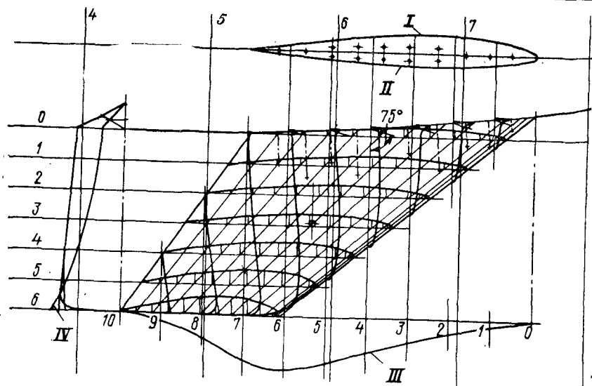
Рис. 15. Теоретический чертеж плавникового киля. I — фланец киля; II — рыбина под 75^\circ к ДП; III — строевая по шпангоутам; IV — строевая по ватерлиниям.
