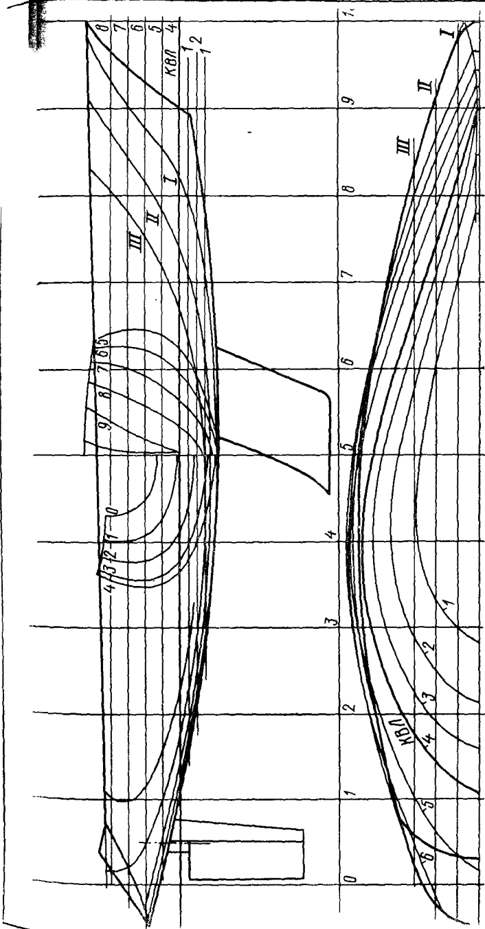
Рис. 40. Теоретический чертеж яхты К. Фелла.
