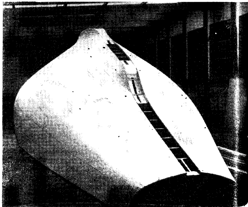
Рис. 78 Болван — положительная форма, на которой строят клееные корпусы. Он стоит примерно в два раза дороже, чем построенный по нему корпус.
