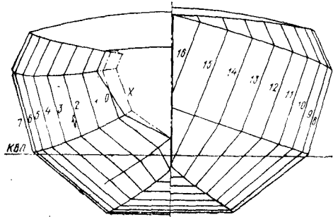
Рис. 59. Теоретический корпус яхты «Гидра».
