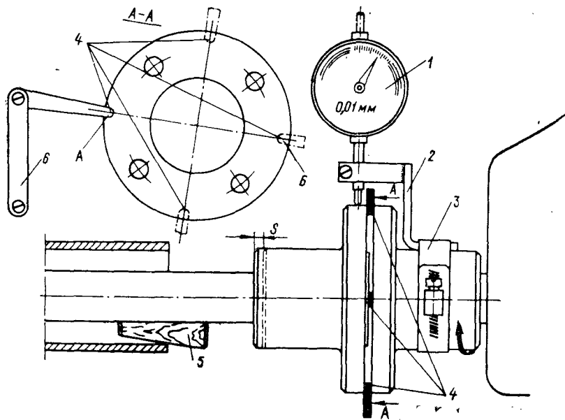
Рис. 178. Схема установки индикатора для контроля смещения линии вала и использования щупа для замера излома. 1—индикатор; 2—держатель индикатора; 3—зажим; 4—точки контроля зазора между фланцами муфты и их несоосности; 5—клин для центровки гребного вала в дейдвудной трубе; 6—щуп.
