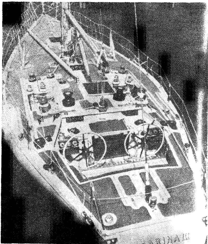
Рис. 176. Палуба яхты «Карина-III» длиной 13,4 м.
