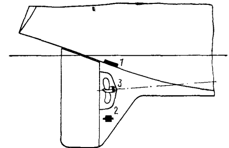
Рис. 203. Расположение защитных анодов на алюминиевой яхте.
