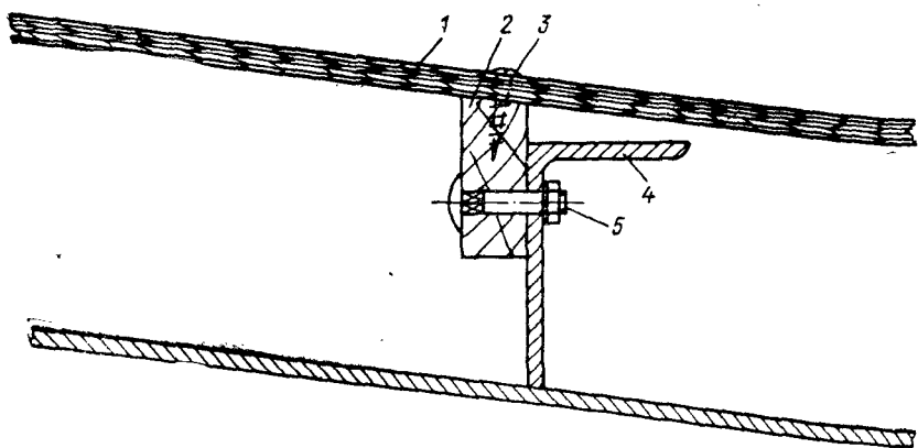
Рис. 149. Узел крепления внутренней зашивки к набору.
