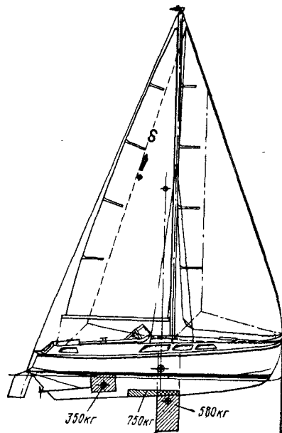
Рис. 20. Остойчивость яхты «Секура» с подъемным килем может быть рассчитана на случай убранного килея точно так же, как для нормального плавания с опущенным килем. Дополнительный внутренний балласт обеспечивает абсолютную остойчивость и при поднятом выдвижном киле.
