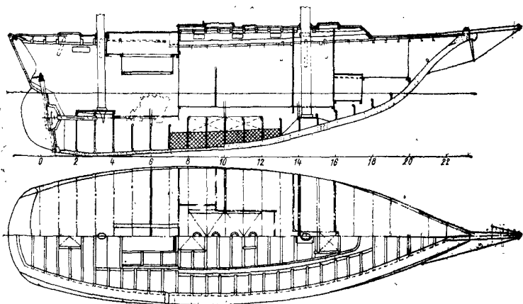
Рис. 109. Конструктивный чертеж кэча из армоцемента.
