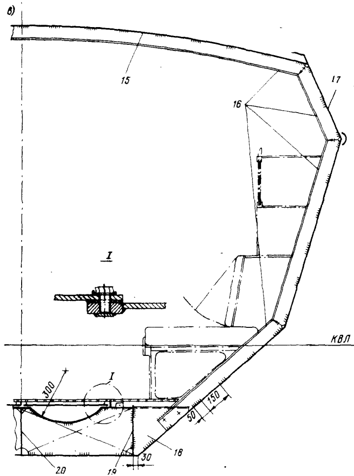
Рис. 4, в. Конструктивный «мидель-шпангоут» стальной яхты «Гндра»: в — рамный шпангоут — шп. 10.
