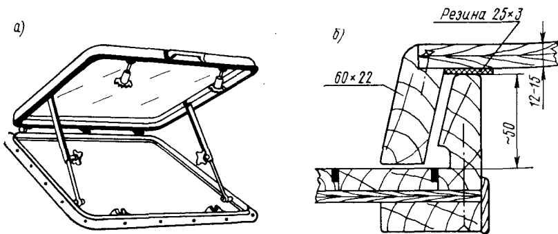
Рис. 152. Конструкция входных люков: а — люк из алюминия и акрилового стекла с минимальным комингсом и резиновым уплотнением; б — деревянный люк с комингсом, образующим водопроток.
