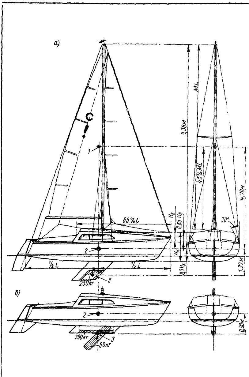
Рис. 18. Схема для оценки остойчивости яхты «Контра» с комплектом нормальных парусов. Центр парусности расположен на расстоянии 45% длины мачты снизу. Масса такелажа рассчитывается детально или взвешиванием (при правильно подобранном такелаже его масса равна
