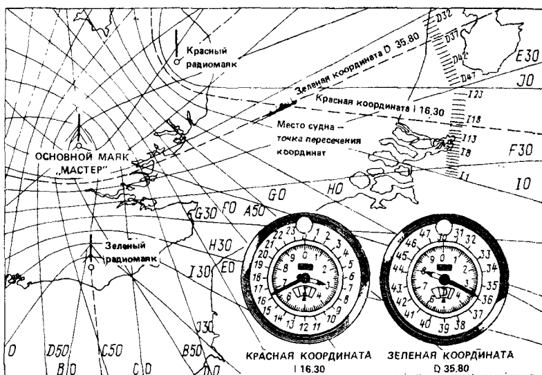
Рис. 191. К определению местоположения судна по навигационной системе «Декка».
