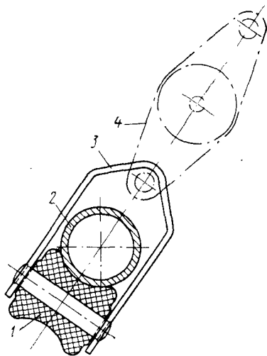
Рис. 158. Простой роликовый ползун на трубчатом поgone. 1—пластмассовый ролик; 2—труба; 3—обойма; 4—блок.
