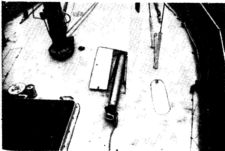
Рис. 165. Труба для хранения спинакер-гика по-походному, вмонтированная в палубу.
