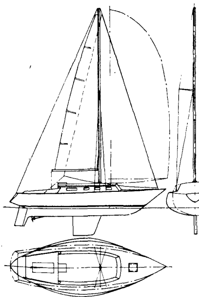
Рис. 23. Проект яхты, созданный по формуле IOR, воспринятый как чрезвычайно «выжиматель формулы» со сверхшироким корпусом. Основные данные: наибольшая длина 11,00 м; длина по КВЛ 8,10 м; ширина 4,00 м; водоизмещение 7,0 т; осадка 1,80 м. Площадь парусности (грот и передний парусный треугольник) 41 \text{ м}^2 ; удельная площадь парусности 1,35. Балл по правилам IOR — около 23 футов.
