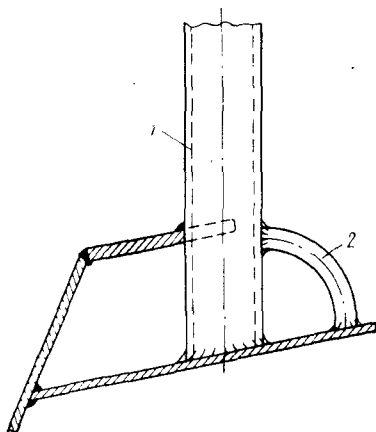
Рис. 156. Крепление леерной стойки на стальной яхте.
