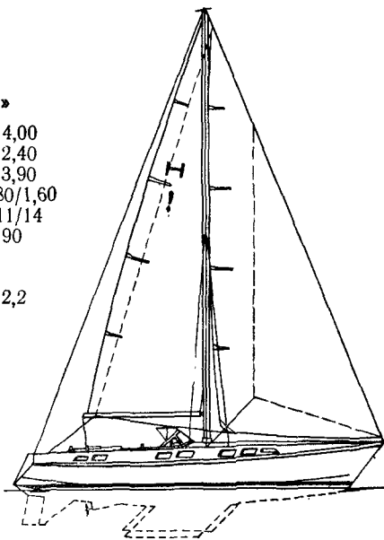
Рис. 57. Схема парусности яхты «Гидра».
