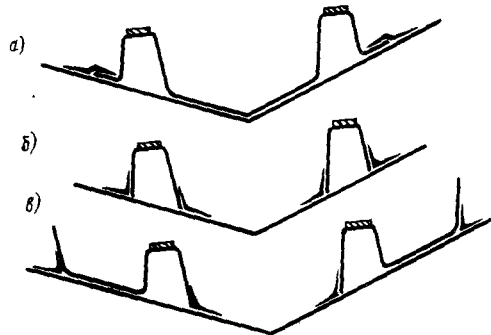
Рис. 128. Поперечные сечения по фундаменту для двигателя.
