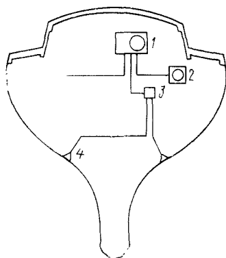
Рис. 183. Принципиальное устройство индикатора эхолота.
