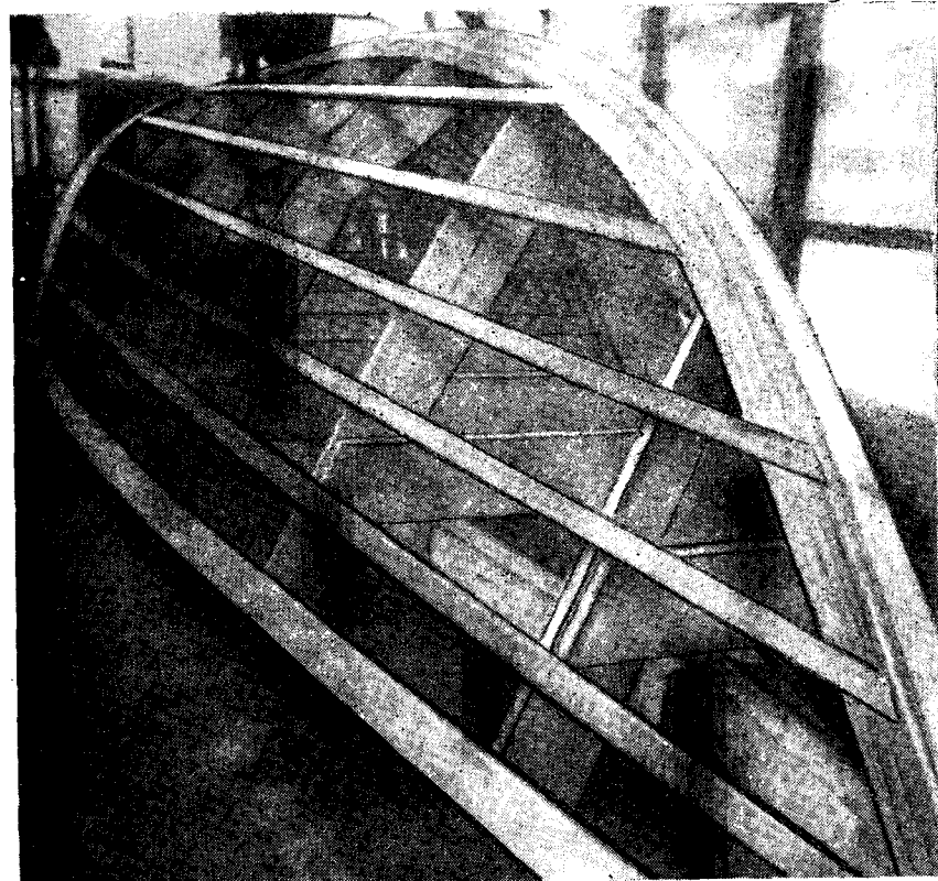
Рис. 76. Стапель-кондуктор для постройки корпуса с диагональной обшивкой.
