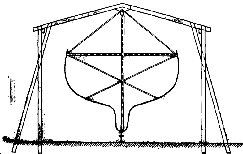
рис. 140. Поперечное сечение стапеля.
