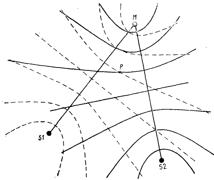
Рис. 193. Упрощенное изображение сети гипербола системы «Лоран». Множество гипербола образуется основной станцией M и двумя вспомогательными S_1 и S_2 . Местонахождение судна P определяется точкой пересечения линий положения двух пар передатчиков.
