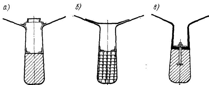
Рис. 130. Балластные кяли.
