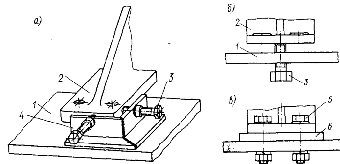
Рис. 179. Приспособление для перемещения двигателя при центровке: а — по горизонтали; б — по вертикали; в — постановка прокладок. 1—опорная плита фундамента; 2—лапа двигателя; 3—отжимной болт; 4—упорное приспособление, приваренное к плите; 5—фундаментный болт; 6—прокладка.
