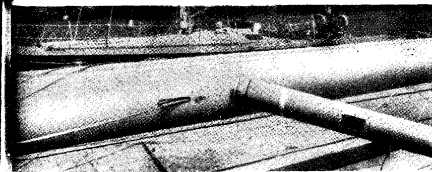
Рис. 160. Крепление основных вант и краспиц на алюминиевой мачте крейсерско-гоночной яхты.
