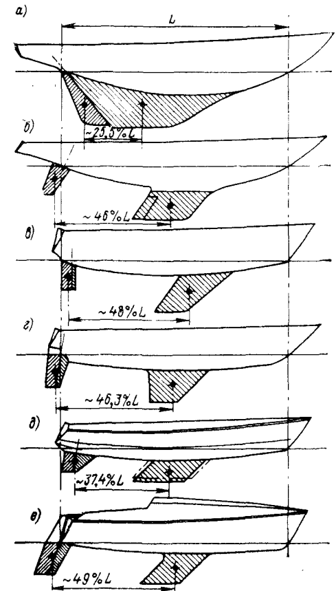
Рис. 14. Сравнительные очертания подводного профиля яхт, условно приведенных к одинаковой длине по ватерлинии L: а — «Индиго»; б — «Оптимист»; в — «Ченс-32»; г — «Христина»; д — «Гидра»; е — «Контра».
