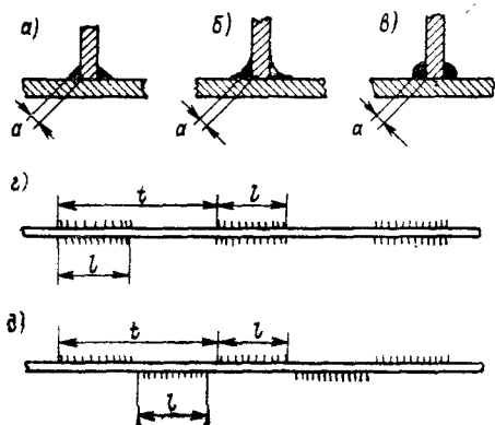
Рис. 89. Элементы угловых швов: а — нормальный шов; б — вогнутый; в — выпуклый; г — шахматный.
