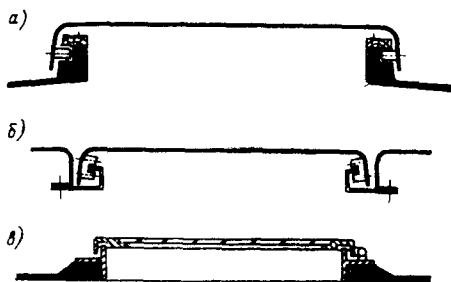
Рис. 132. Люки: сдвижной ( а и б ) и откидной светлый ( в ).
