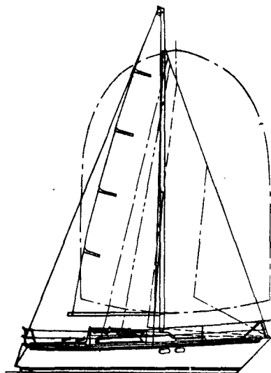
Рис. 26. Схема парусности яхты «Пион»: грот — 19 м 2 ; генуя № 1 — 28,9 м 2 ; генуя № 2 — 24,7 м 2 ; стаксель № 1 — 18,6 м 2 ; стаксель № 2 — 12,5 м 2 ; штормовой стаксель — 6,4 м 2 ; толбач — 12,1 м 2 ; спинакер — 62 м 2 ; ричель — 29,1 м 2 .
