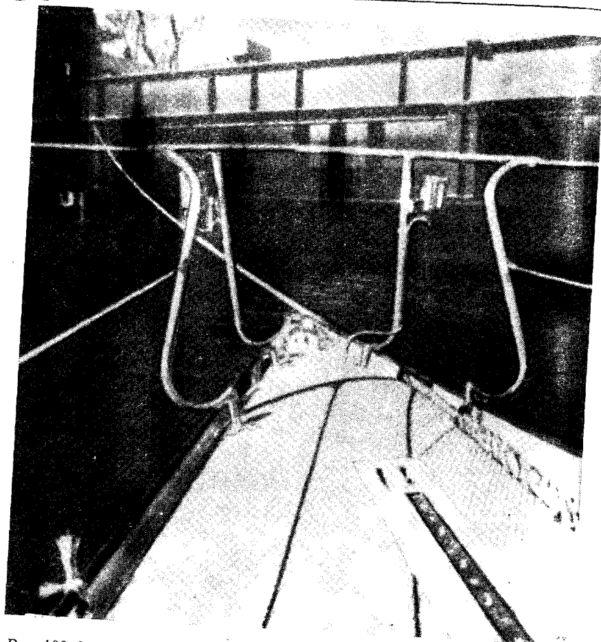
Рис. 166. Носовой релинг, приспособленный для крепления по-ходному двух спинакер-гиков.
