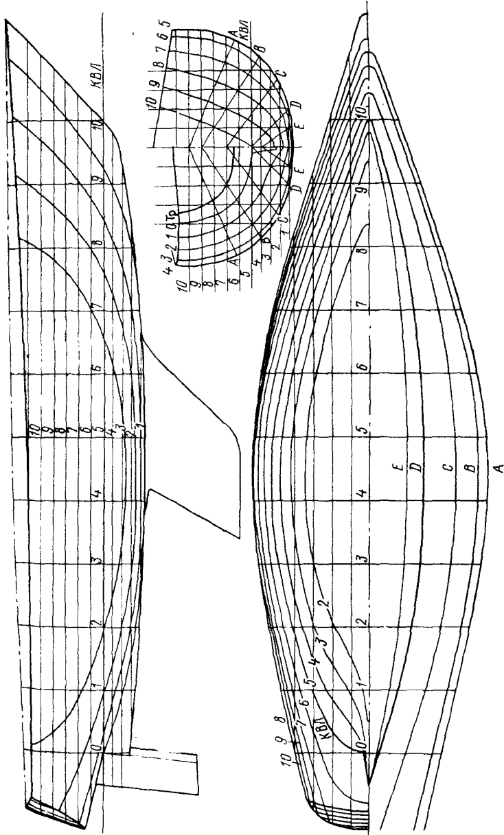
Рис. 33 Теоретический чертеж яхты «Спанкер».
